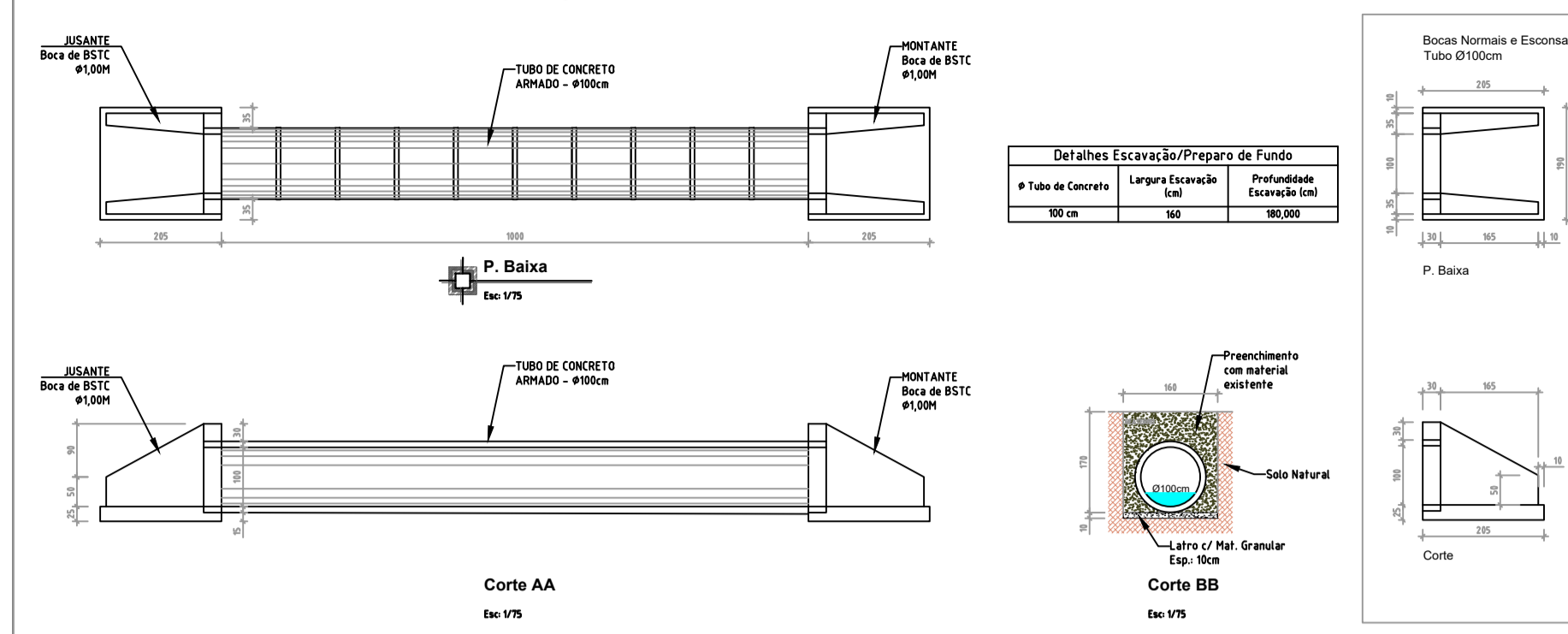
Meta 10: Restabelecimento de sistema de drenagem pluvial na comunidade de Linha Nona
