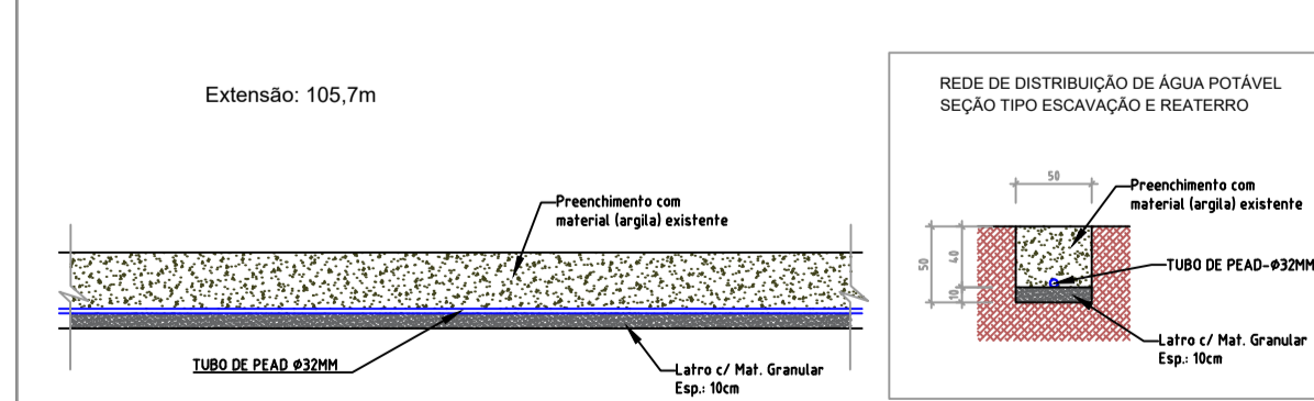
Meta 19: Restabelecimento de rede de água potável na comunidade Linha Sétima São Roque
