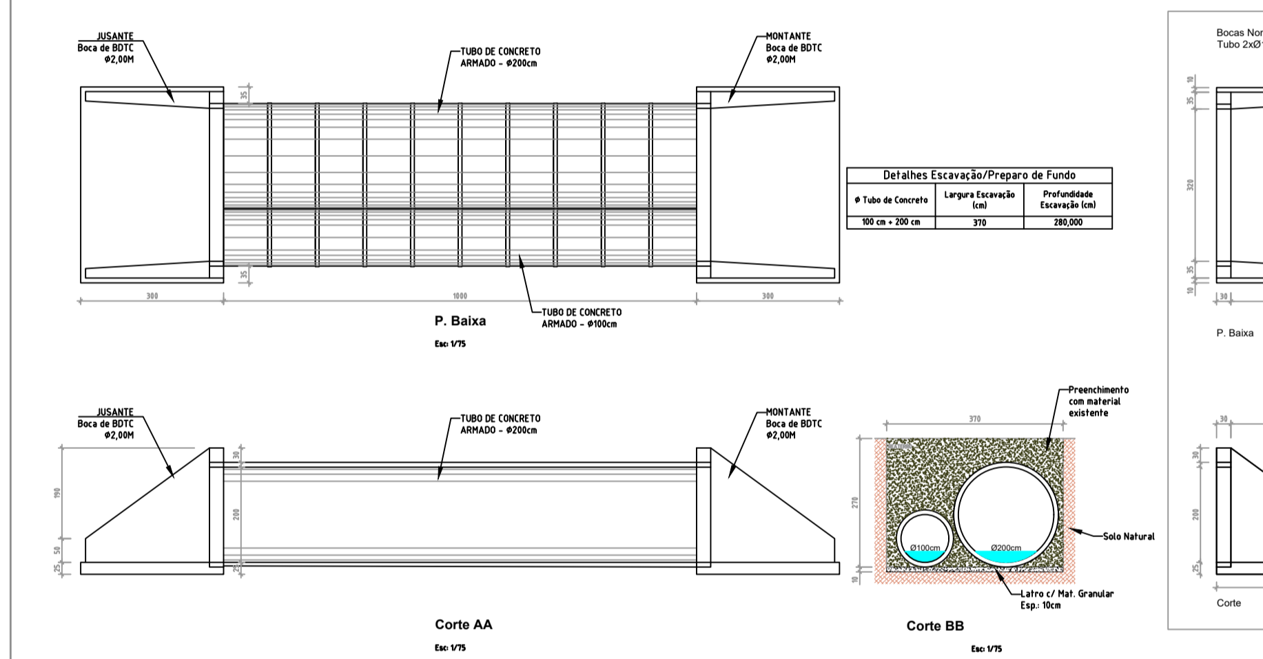
Meta 16: Restabelecimento de sistema de drenagem pluvial na comunidade de Linha Sétima Zanette
