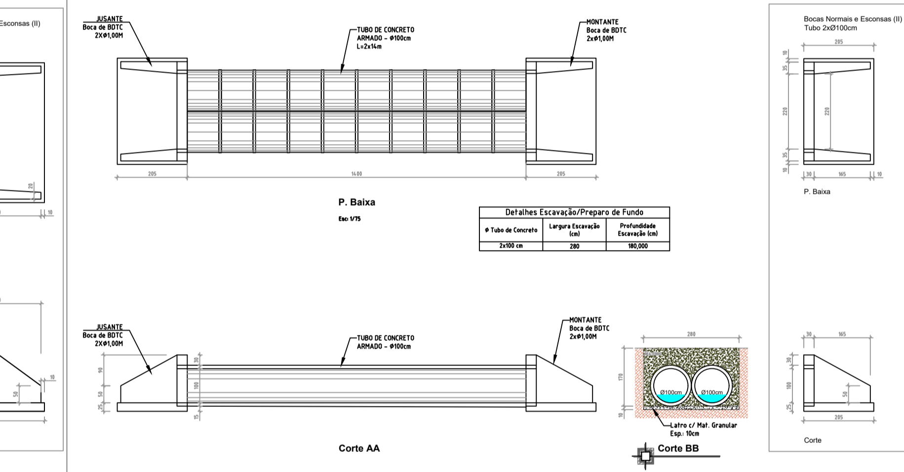
Meta 14: Restabelecimento de sistema de drenagem pluvial na comunidade de Linha Nona Mioto
