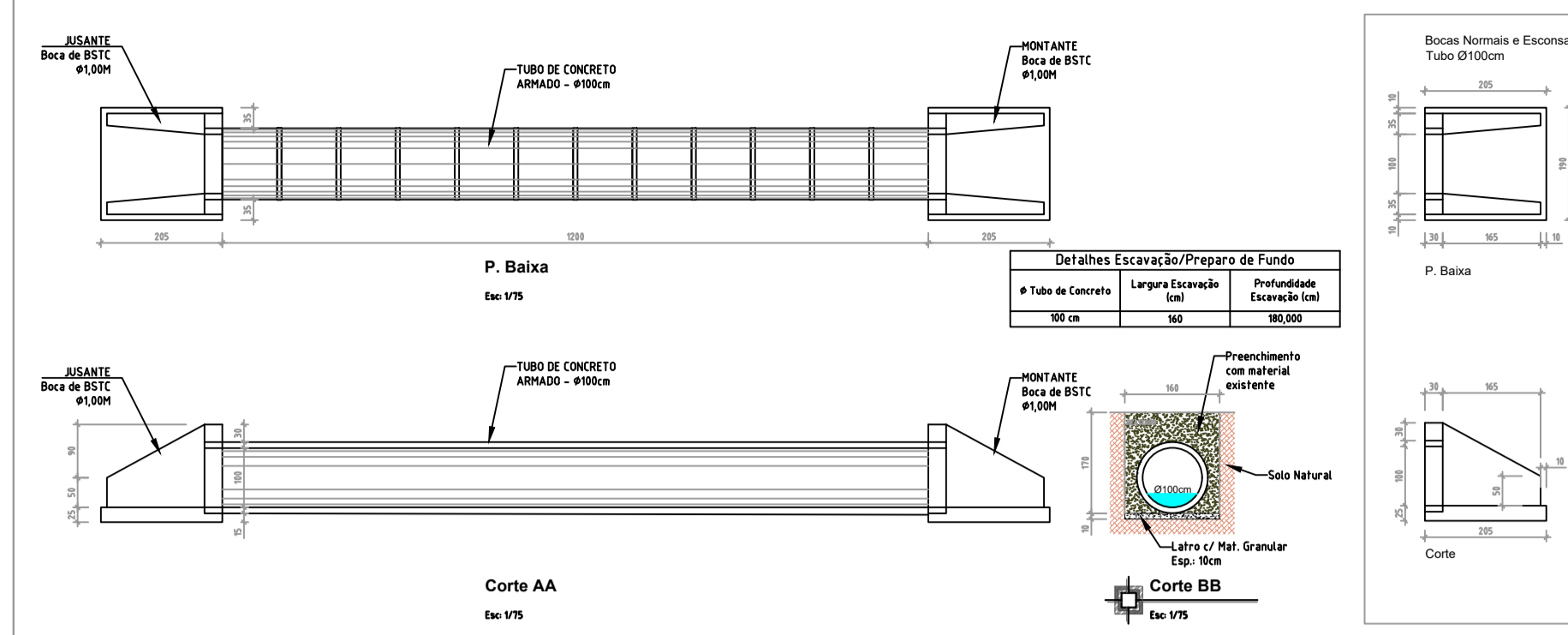
Meta 11: Restabelecimento de sistema de drenagem pluvial na comunidade de Linha Coxilha Seca
