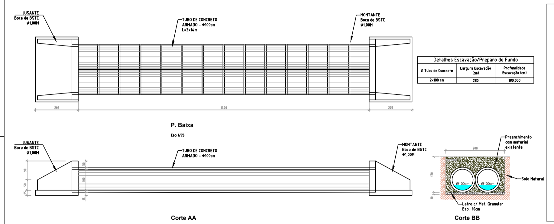
Meta 13: Restabelecimento de sistema de drenagem pluvial na comunidade de Linha Nona Último
