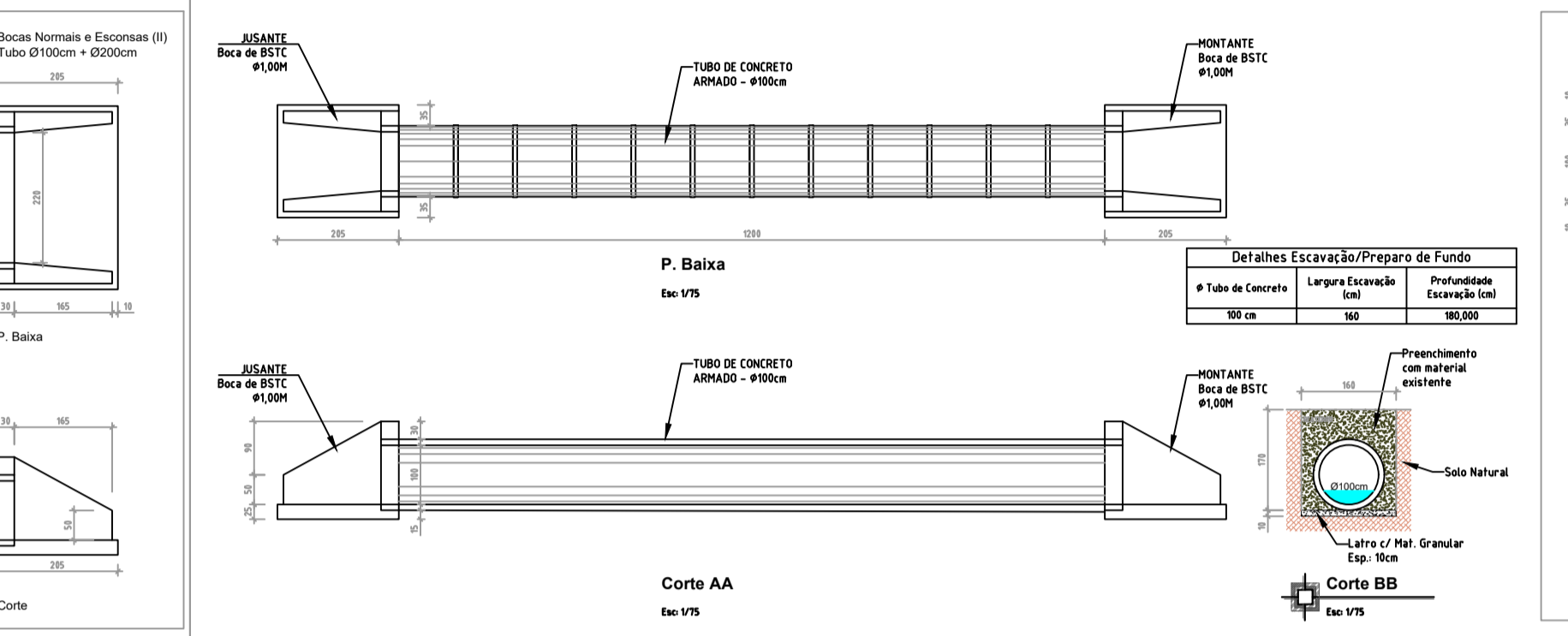
Meta 14: Restabelecimento de sistema de drenagem pluvial na comunidade de Linha Nona Mioto
