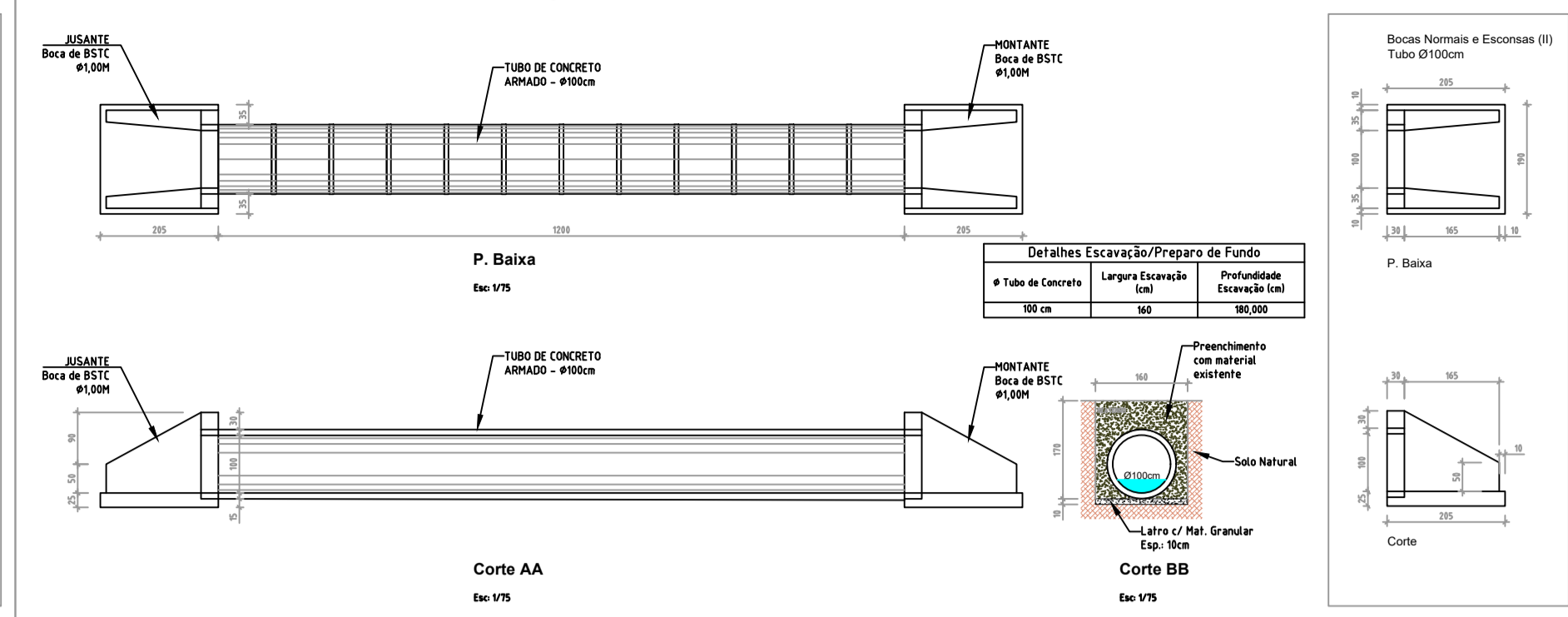
Meta 12: Restabelecimento de sistema de drenagem pluvial na comunidade de Linha Nona Passagem
