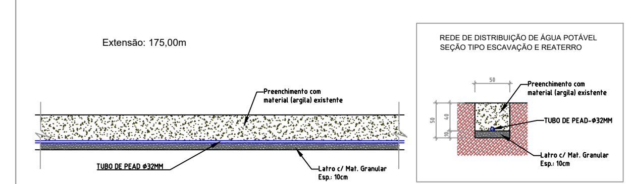
Meta 20: Restabelecimento de rede de água potável na comunidade Linha Nona
