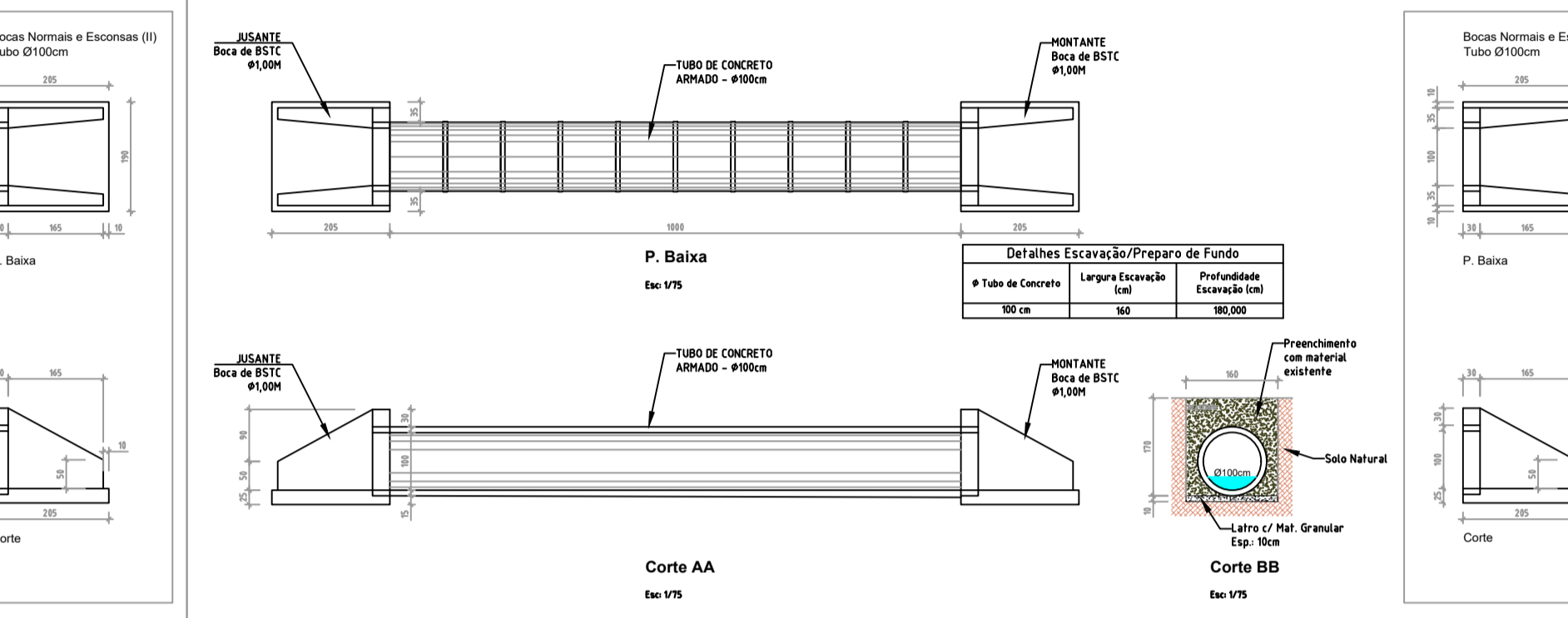
Meta 15: Restabelecimento de sistema de drenagem pluvial na comunidade de Linha Sétima
